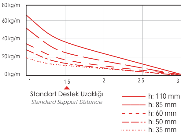
ETT Serisi Yükleme Diyagramı (ETT Series Loading Diagram)
