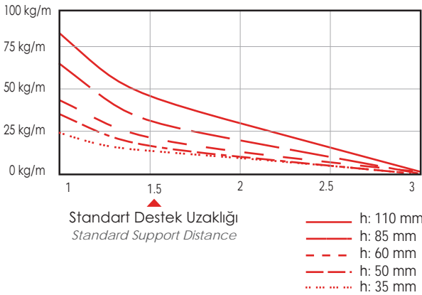
ETT Serisi Yükleme Diyagramı (ETT Series Loading Diagram)
