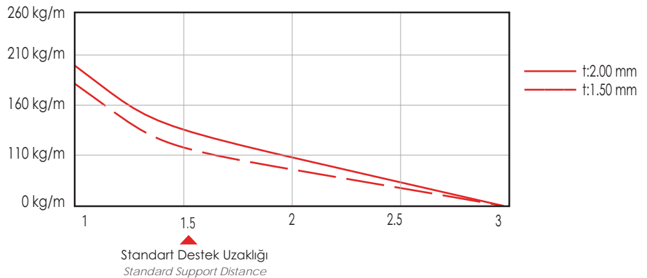
EL50 Serisi Yükleme Diyagramı (EL50 Series Loading Diagram)
