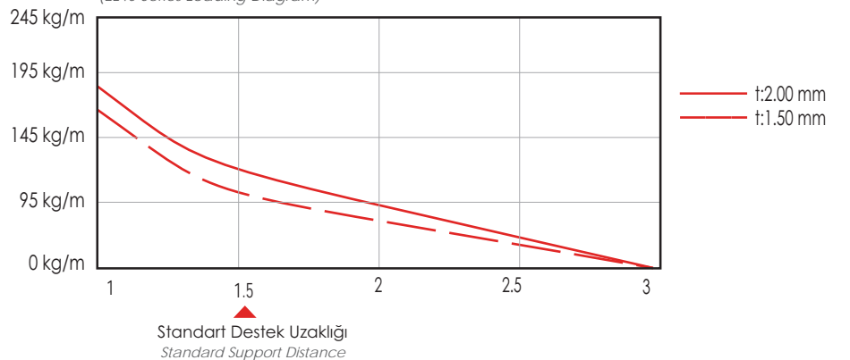
EL40 Serisi Yükleme Diyagramı (EL40 Series Loading Diagram)
