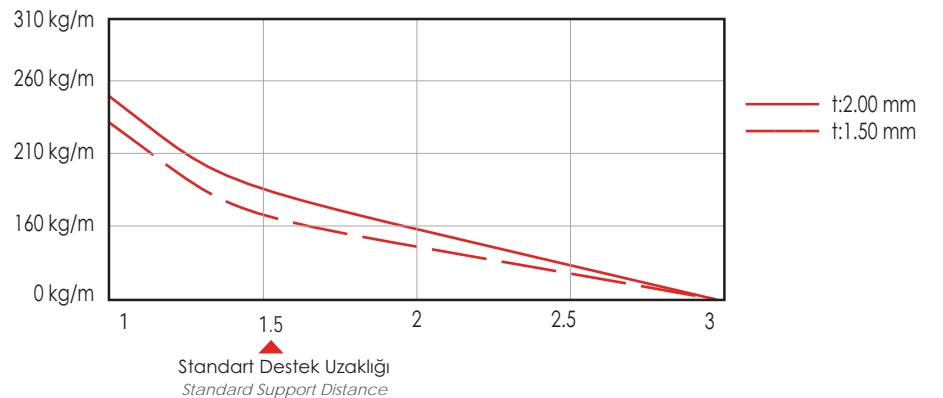
EL100 Serisi Yükleme Diyagramı (EL100 Series Loading Diagram)
