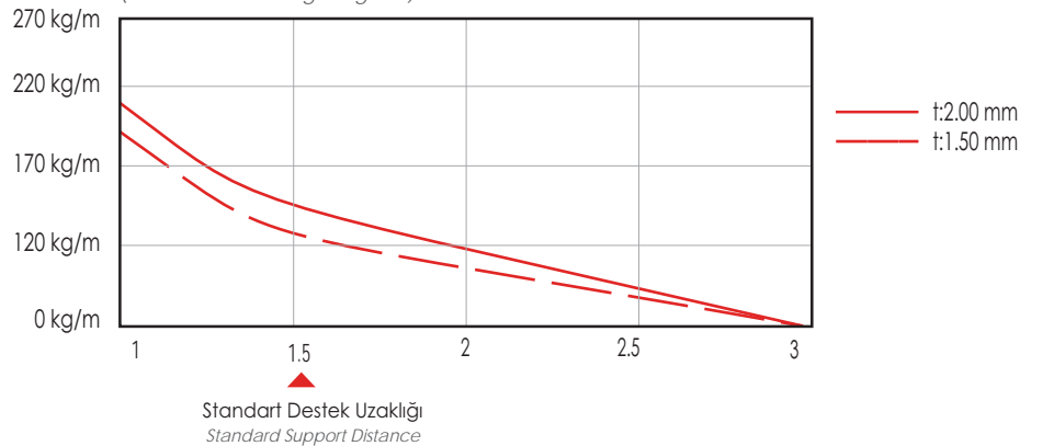
EL60 Serisi Yükleme Diyagramı (EL60 Series Loading Diagram)
