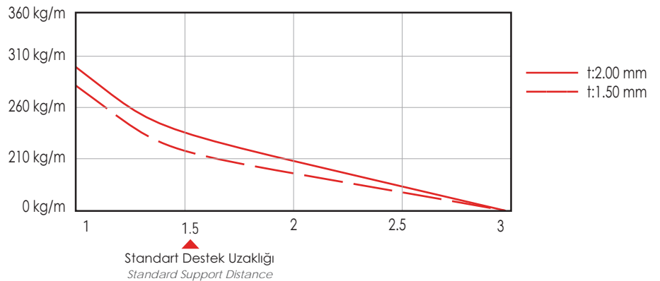
EL150 Serisi Yükleme Diyagramı (EL150 Series Loading Diagram)
