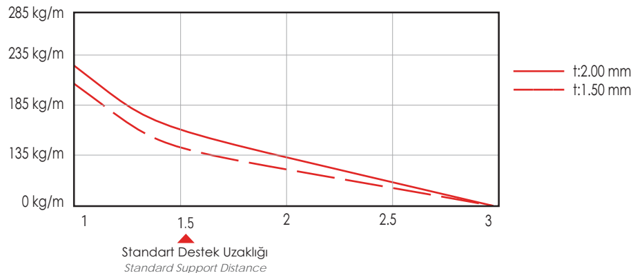
EL75 Serisi Yükleme Diyagramı (EL75 Series Loading Diagram)
