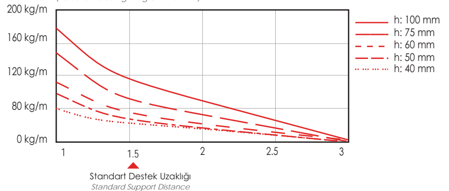
EU Serisi Yükleme Diyagramı - t:1 mm (EU Series Loading Diagram - t:1mm)
