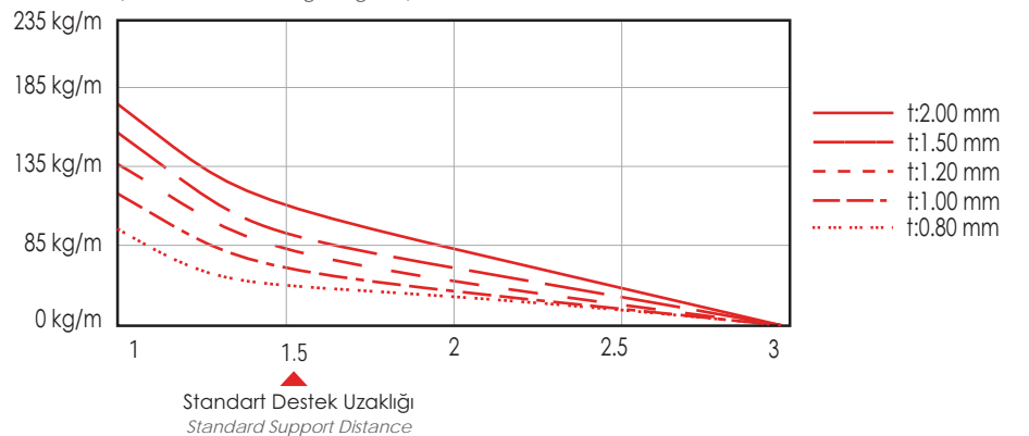
EH40 Serisi Yükleme Diyagramı (EH40 Series Loading Diagram)
