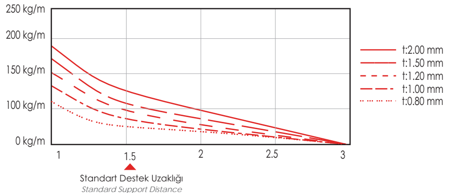
EH50 Serisi Yükleme Diyagramı (EH50 Series Loading Diagram)
