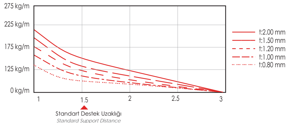
EH75 Serisi Yükleme Diyagramı (EH75 Series Loading Diagram)
