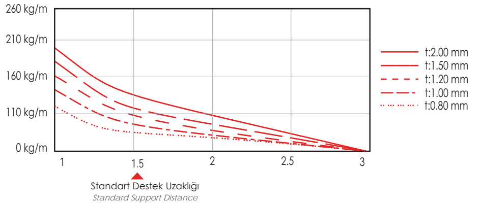
EH60 Serisi Yükleme Diyagramı (EH60 Series Loading Diagram)
