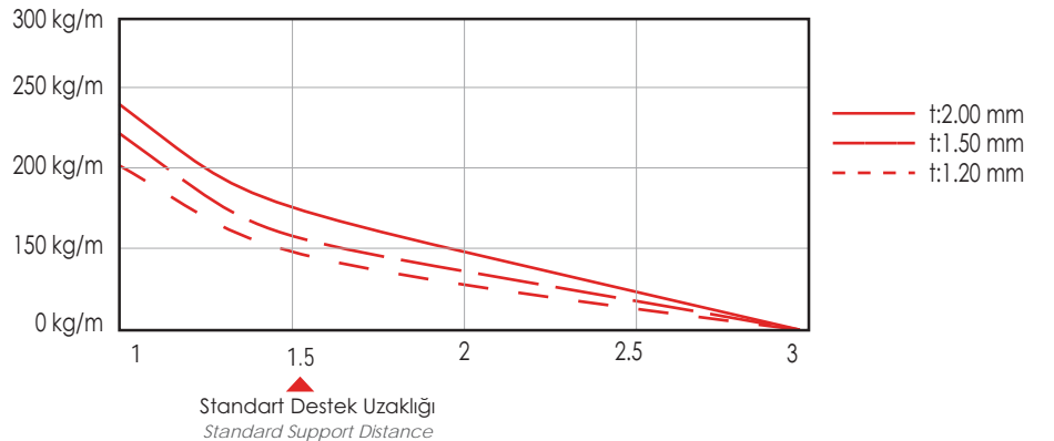
EH100 Serisi Yükleme Diyagramı (EH100 Series Loading Diagram)
