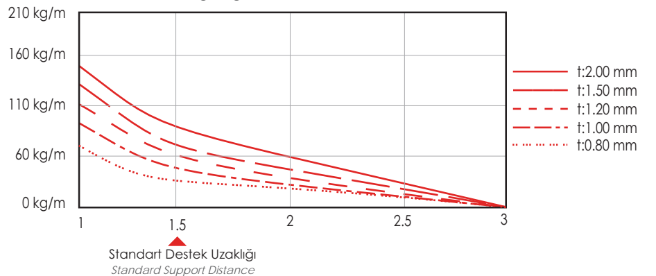
EN40 Serisi Yükleme Diyagramı (EN40 Series Loading Diagram)
