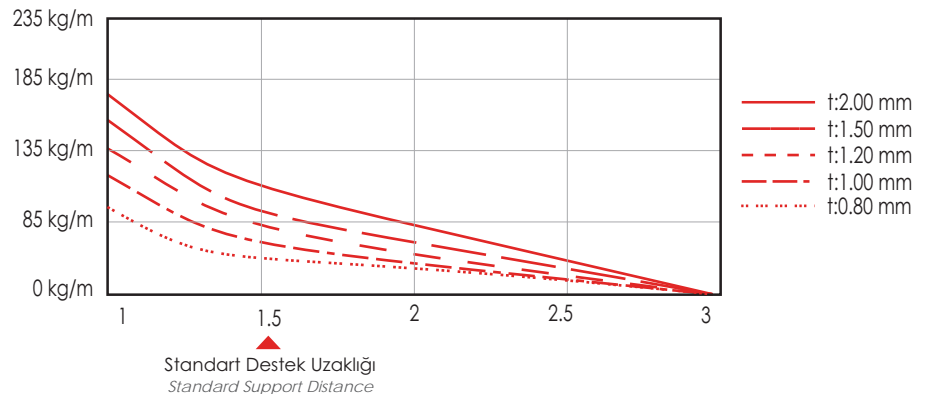
EN60 Serisi Yükleme Diyagramı (EN60 Series Loading Diagram)
