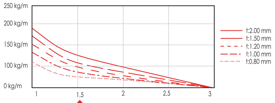
EN75 Serisi Yükleme Diyagramı (EN75 Series Loading Diagram)
