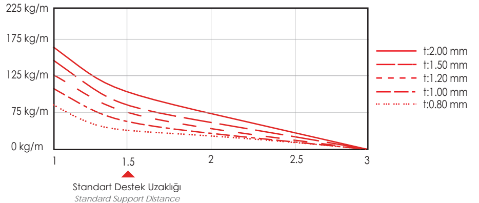
EN50 Serisi Yükleme Diyagramı (EN50 Series Loading Diagram)
